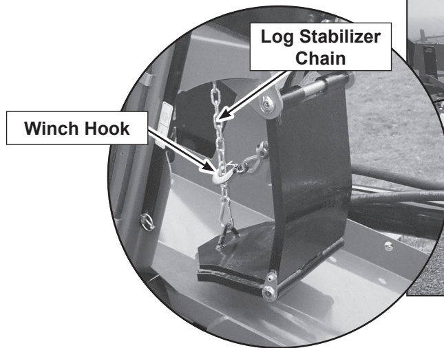
Fig. 16 LOG CHUTE
