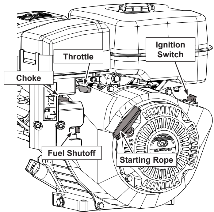
Fig. 4 CONTROLS: WP630: SUBARU EX27 9HP
