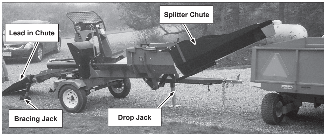
Fig. 16 LOG CHUTE
