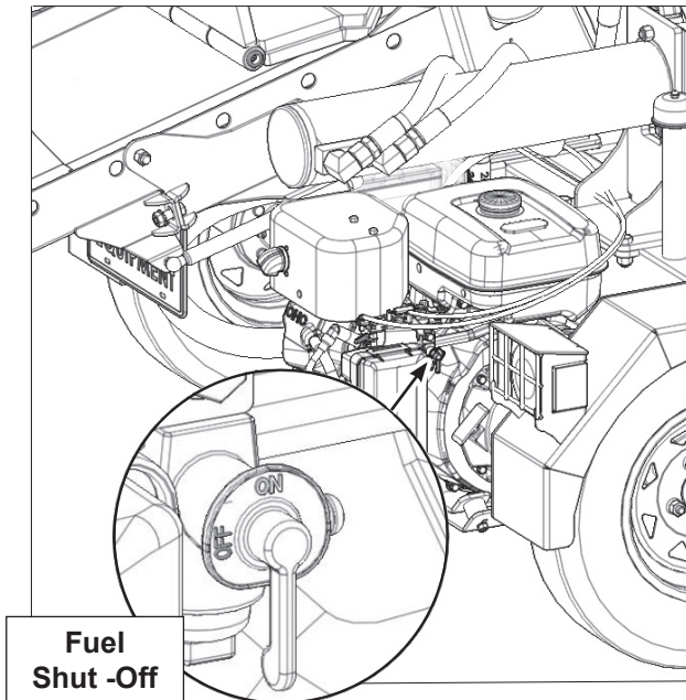
Fig. 3 WP830 & WP860: SUBARU EX40 14HP
