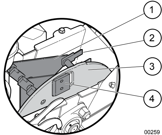
Fig. 47 – Rotor
