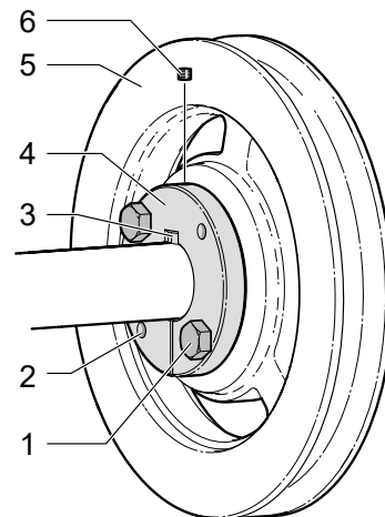
Fig. 46 —Rotor Sheave
