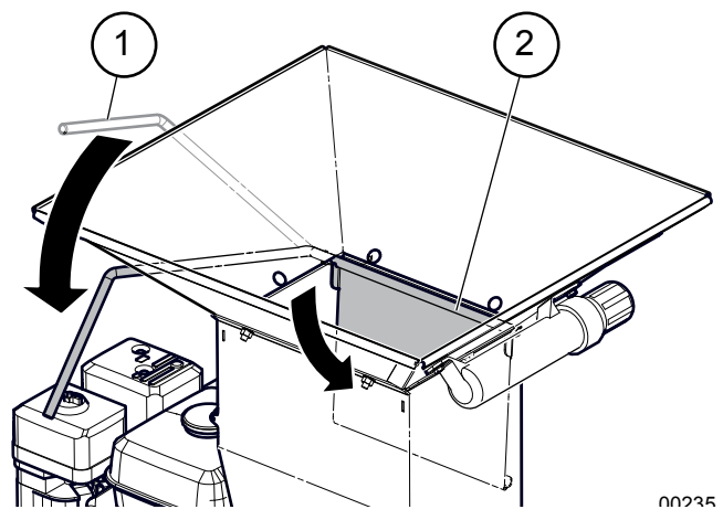
Fig. 13–Shredder Hopper Flap
