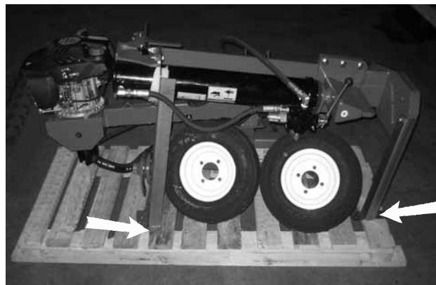
Supports installés pour le transport (longeron de la fendeuse)
