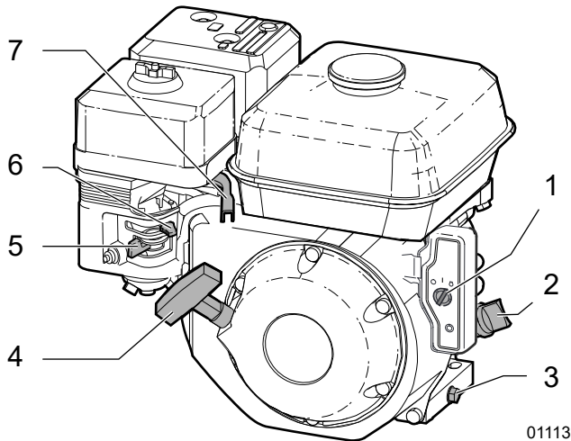
Fig. 6 – Commandes du moteur
