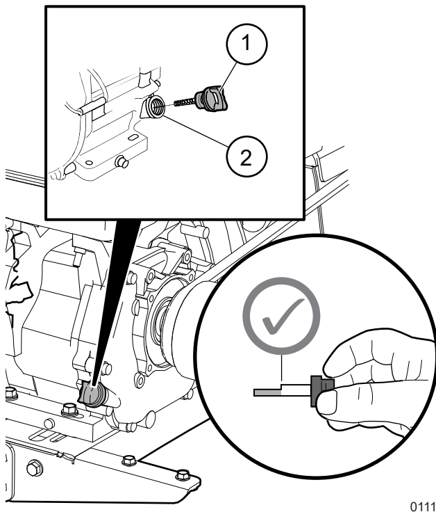
Fig. 18—Vérification du niveau d'huile moteur
