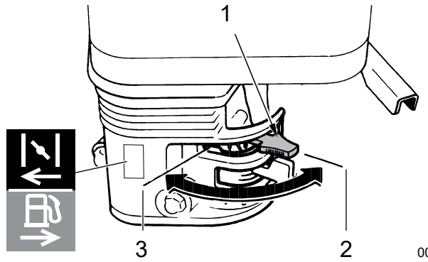
Fig. 20 – Manette d'étrangleur
