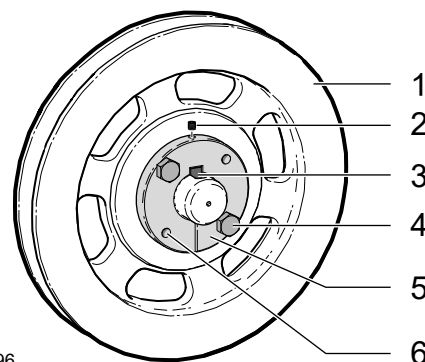
Fig. 39 – Poulie du rotor
