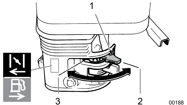
Fig. 8 – Manette d'étrangleur
