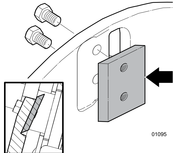
Fig. 41 – Arête tranchante de la lame du rotor vers l'extérieur
