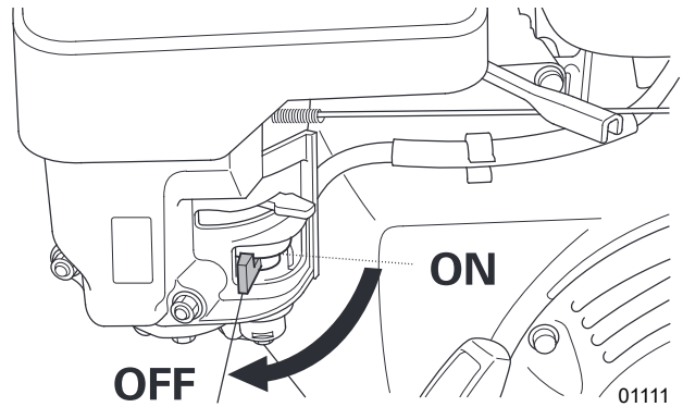
Fig. 25 – Vanne de combustible
