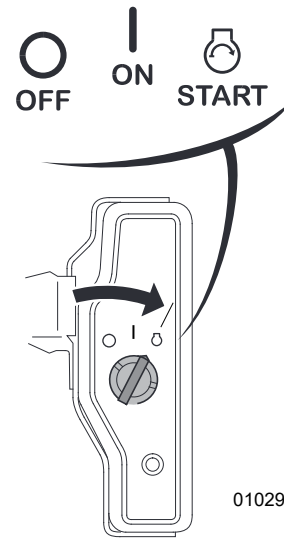
Fig. 7 – Interrupteur de démarrage du modèle BXMT3213
