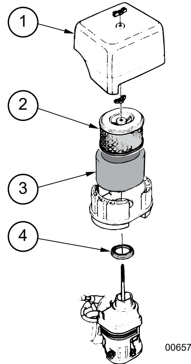
Fig. 32 – Assemblage du purificateur d'air
