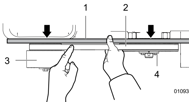
Fig. 35 —Alignement de la courroie d'entraînement
