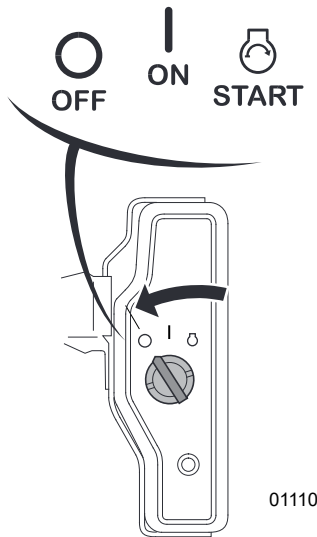
Fig. 24 – Interrupteur de démarrage
