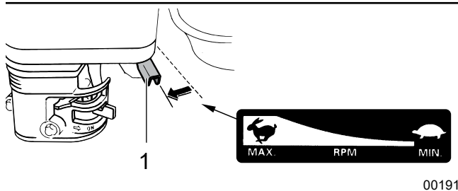
Fig. 10 – Positions de la manette de commande des gaz
