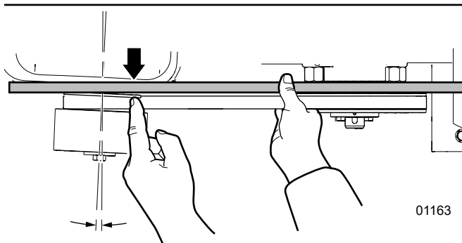
Fig. 36 – Désalignement du support du moteur
