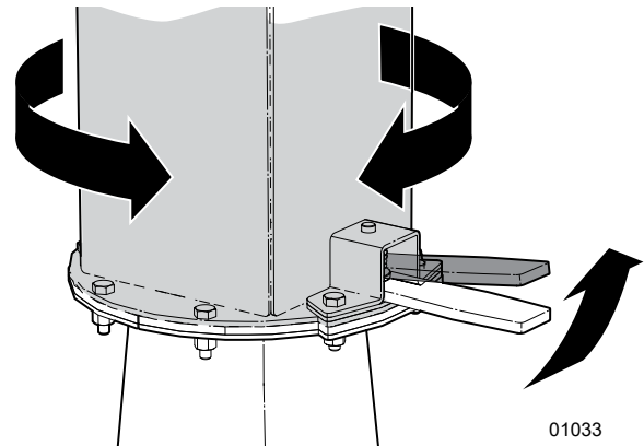
Fig. 15–Rotation de la goulotte de décharge
