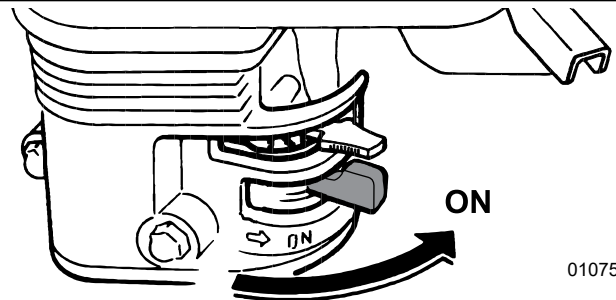
Fig. 19—Manette de la vanne de combustible
