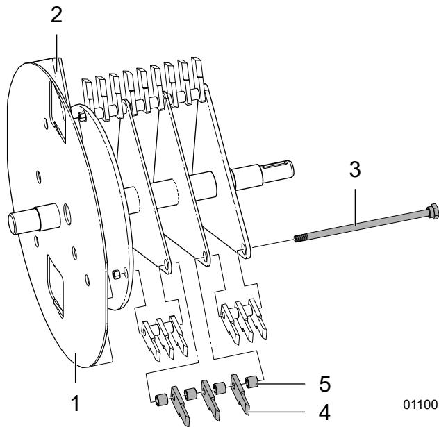
Fig. 44—Assemblage du rotor
