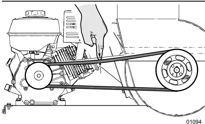
Fig. 34 —Tension de la courroie d'entraînement du rotor
