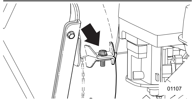
Fig. 29 – Boulon supérieur du boîtier du rotor
