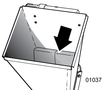
Fig. 27 – Rideau de sécurité de la trémie d'alimentation
