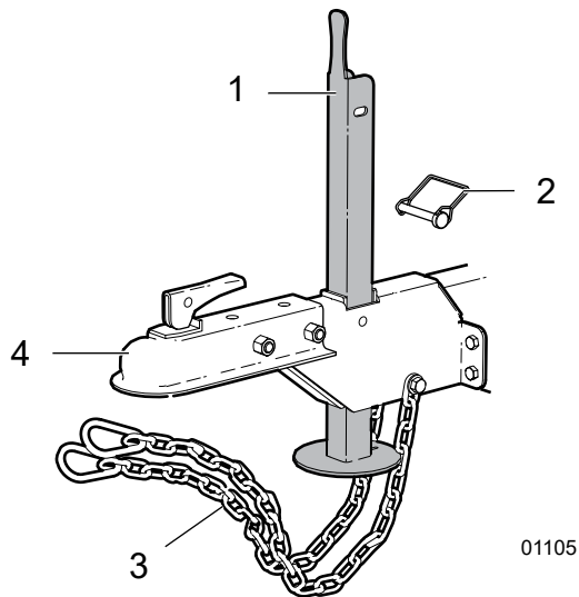
Fig. 14–Coupleur d'attelage
