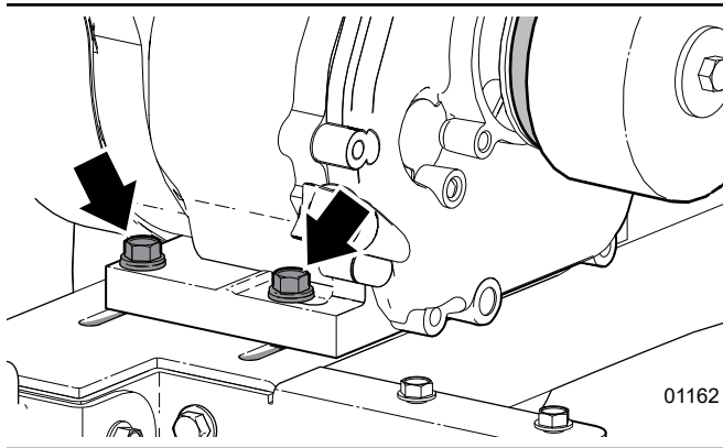
Fig. 37 – Boulons d'installation du moteur
