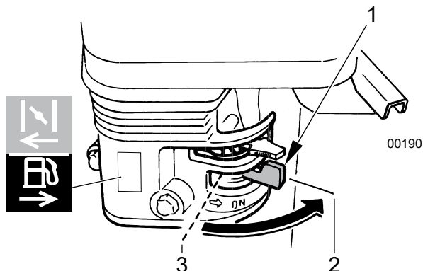
Fig. 9 – Manette de la vanne de combustible
