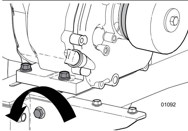
Fig. 33 —Boulon de réglage de la tension de la courroie d'entraînement
