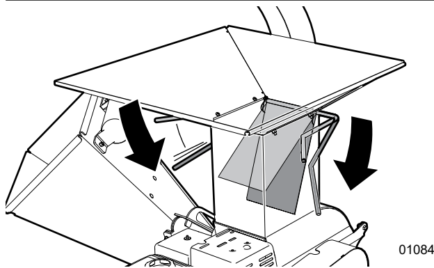
Fig. 12 – Leviers de l'obturateur d'alimentation
